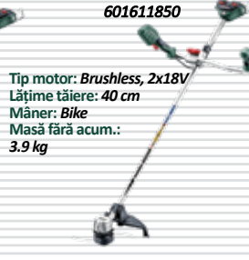
Motocoasă FSB 36-18 LTX BL40 601611850
